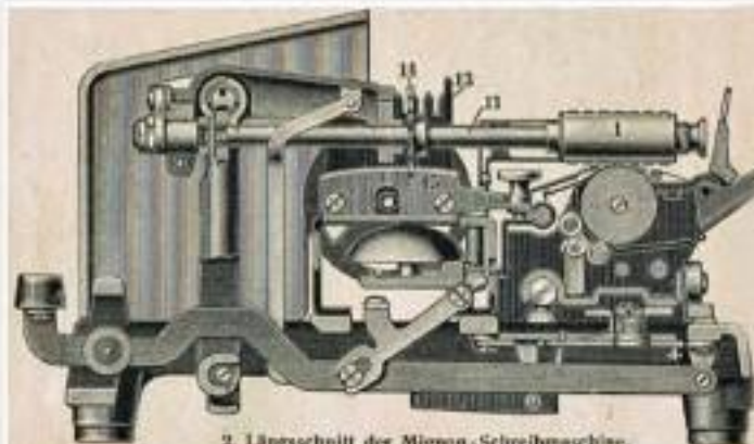
2. Längsschnitt der Mignon-Schreibmaschine.
